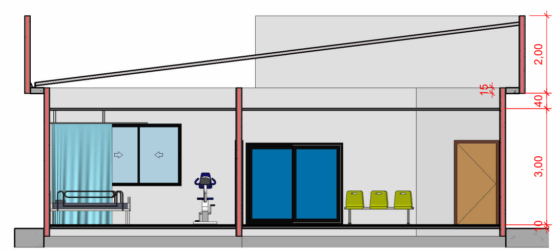
8 CORTE AA 1 : 100
