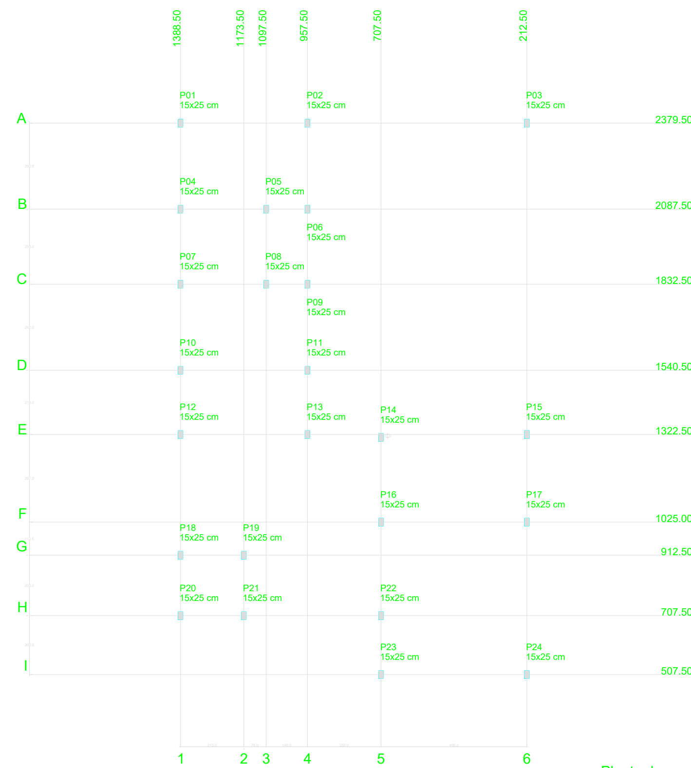
Planta de cargas escala 1:50
