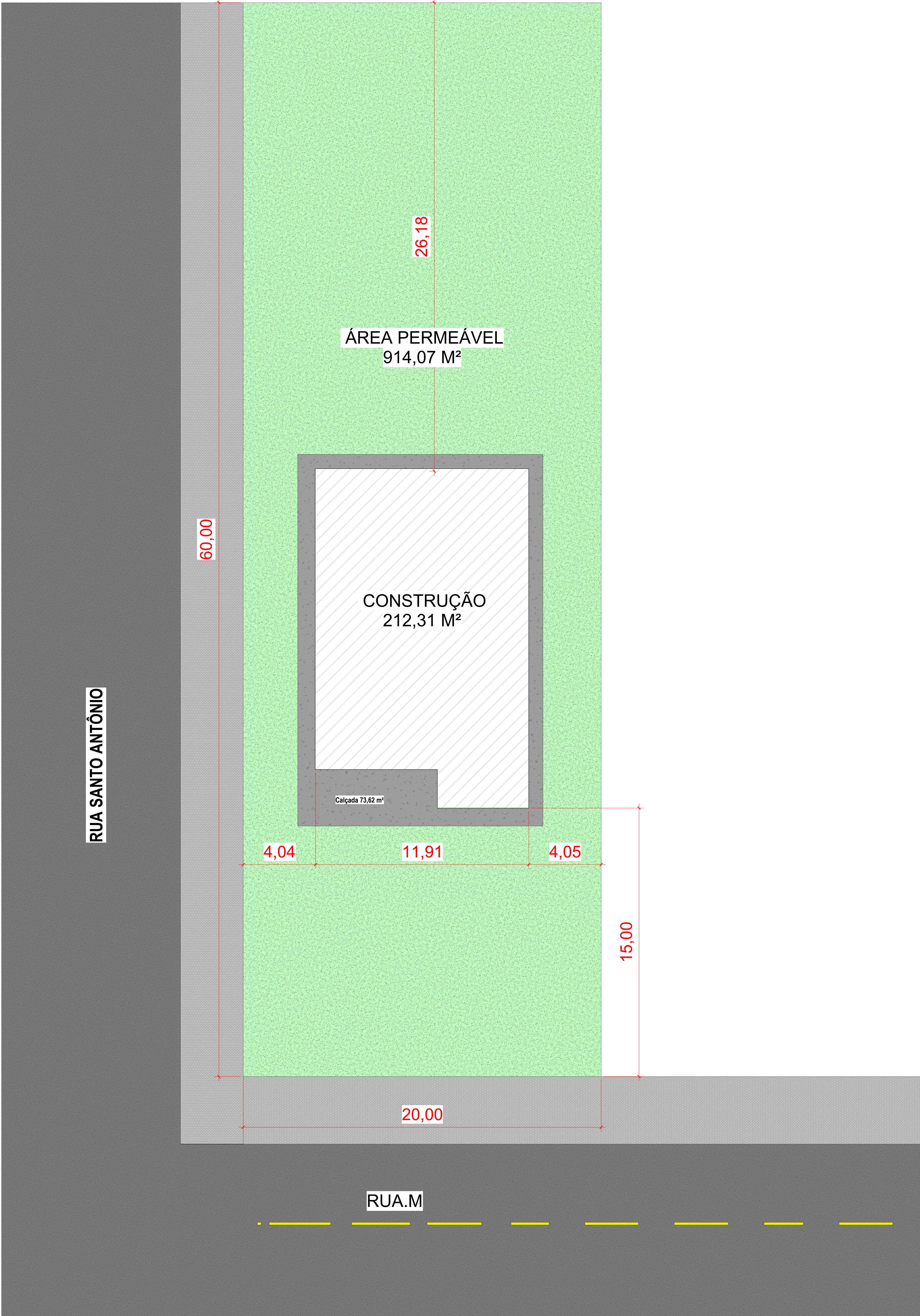
3 Planta de locação 1 : 100
