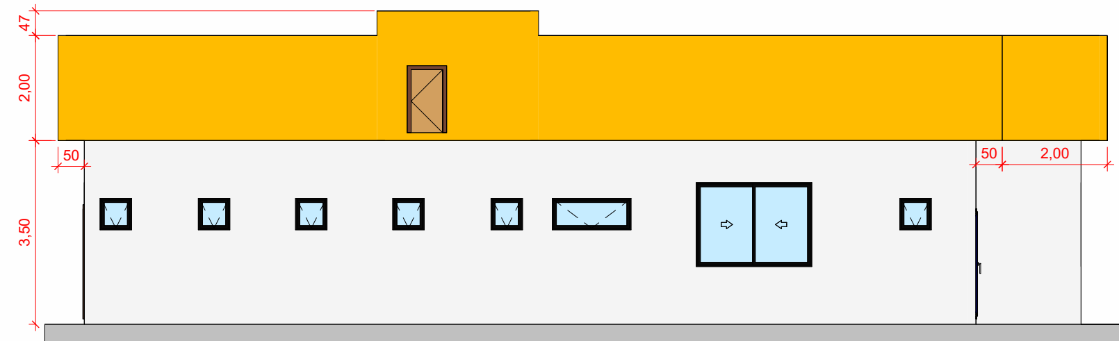
6 FACHADA LATERAL ESQUERDA 1 : 100
