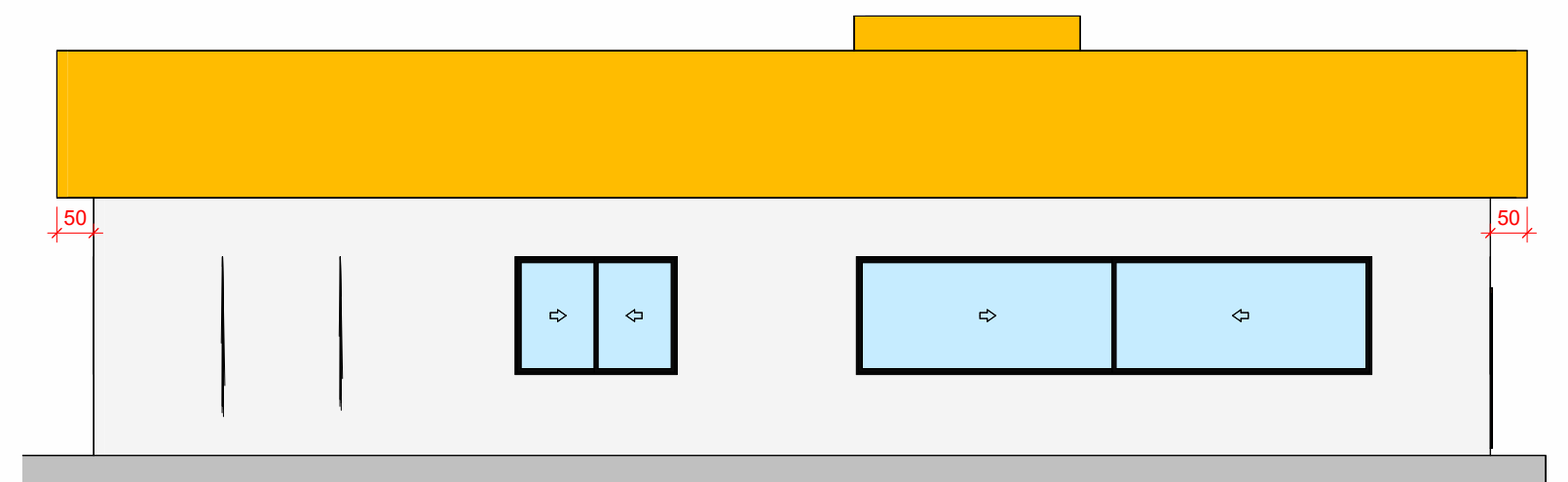
7 FACHADA LATERAL DIREITA 1 : 100
