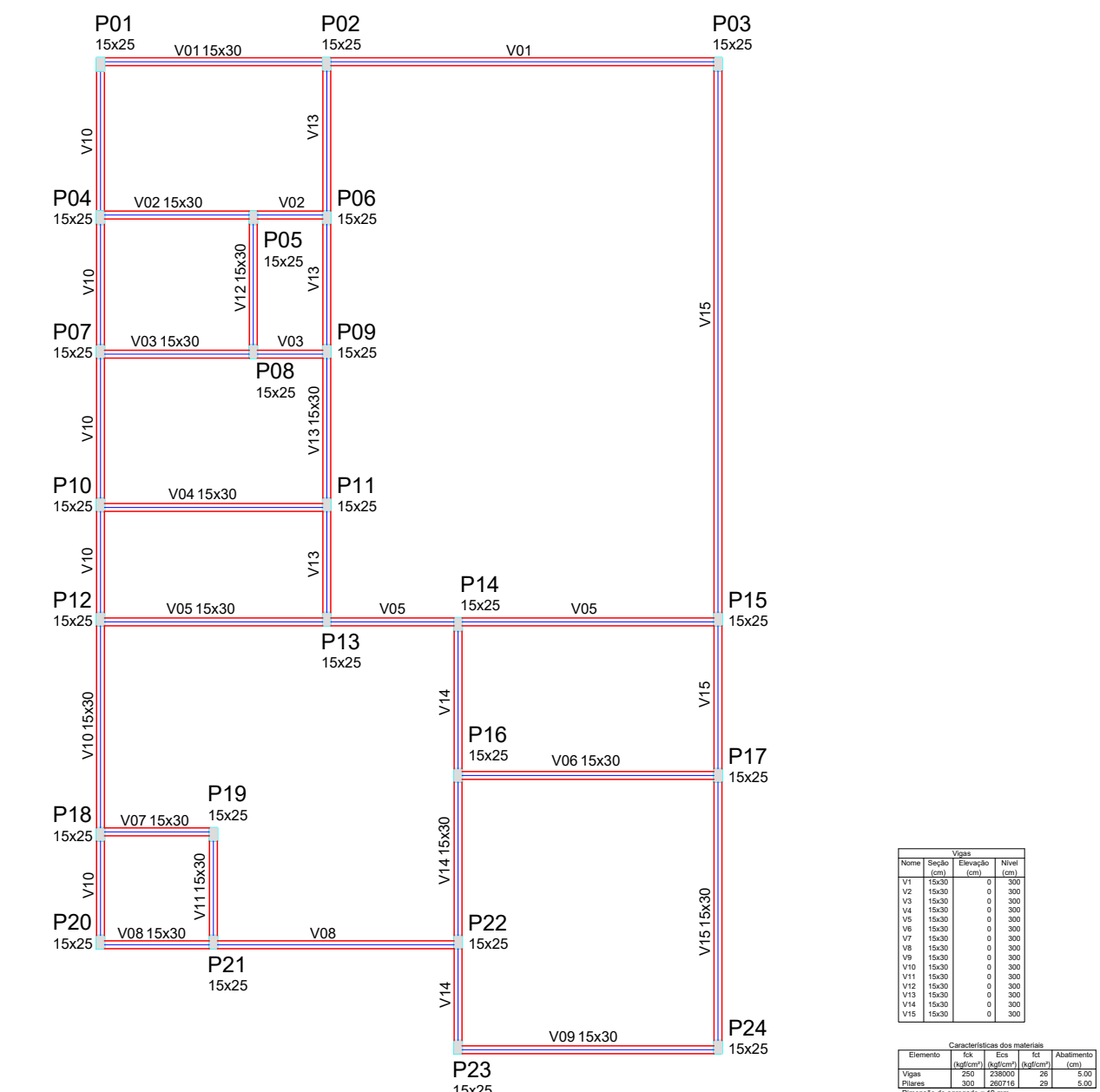
Forma do pavimento de Infraestrutura escala 1:50
