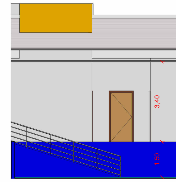
10 CORTE CC 1 : 100
