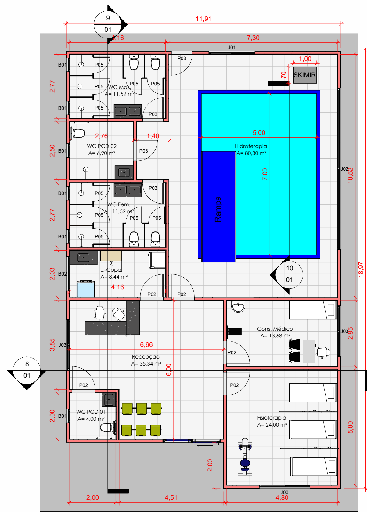
1 PLANTA BAIXA 1 : 100
