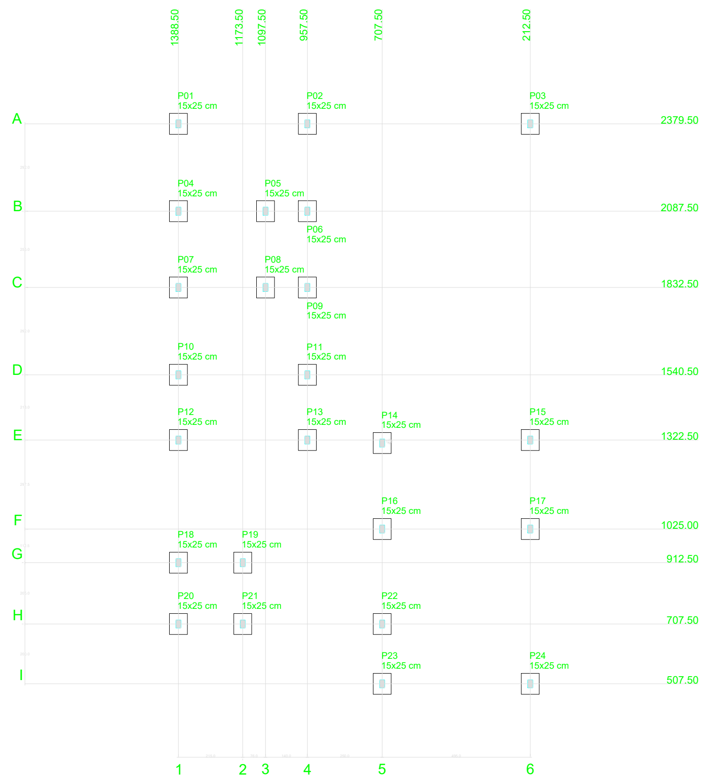
Planta de localização escala 1:50
