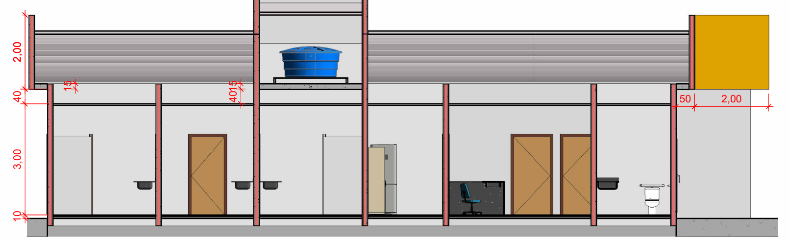
9 CORTE BB 1 : 100
